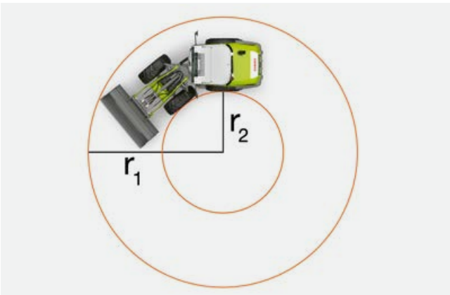
Angegebene Werte gültig für Bereifung Dunlop 365 / 70 R 18 (TORION 535) bzw. Dunlop 365 / 80 R 20 (TORION 639)
