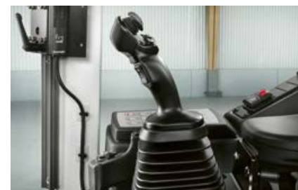
Die automatische Schaufelrückführung lässt sich per Knopfdruck am Joystick aktivieren.
