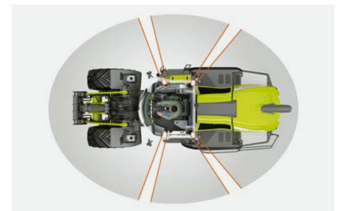
360°-Sicht durch abgerundete Frontscheibe
