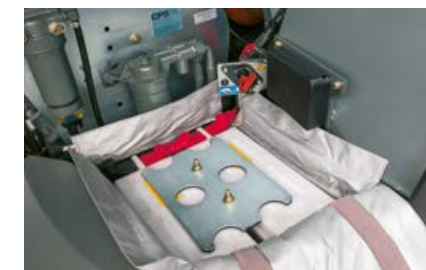
Batterie und Hauptschalter des TORION 1511-1177 sind problemlos zugänglich.
