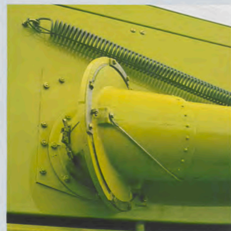
Korndichtes Auslaufrohr
