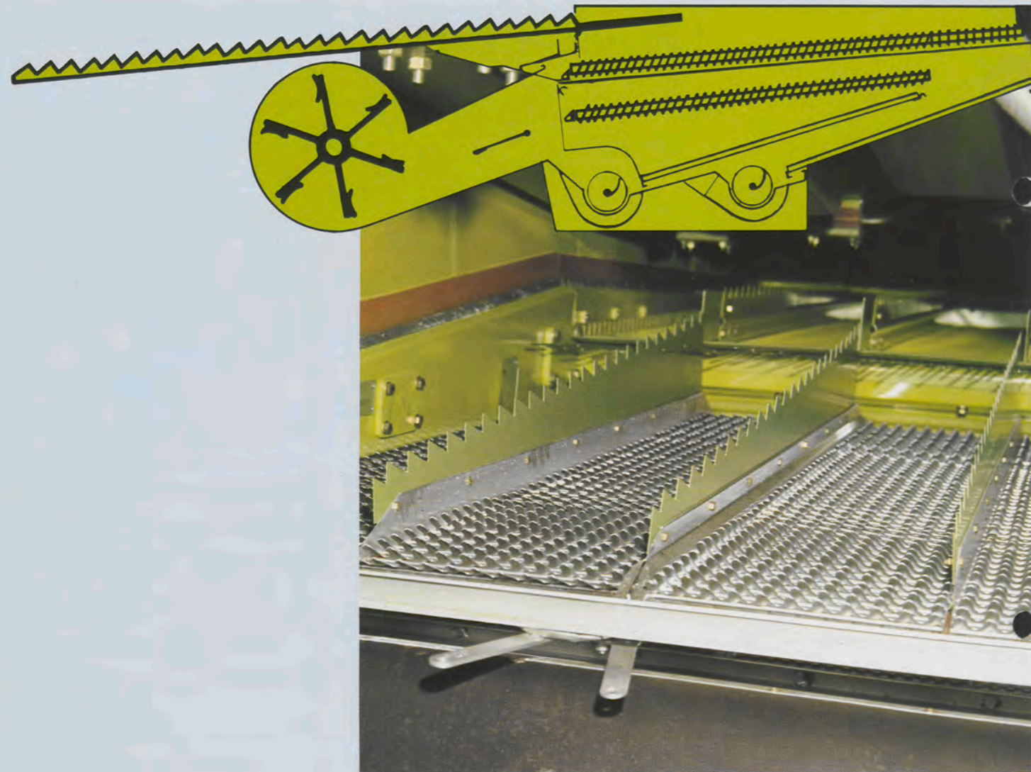
Große Reinigungsflächen
