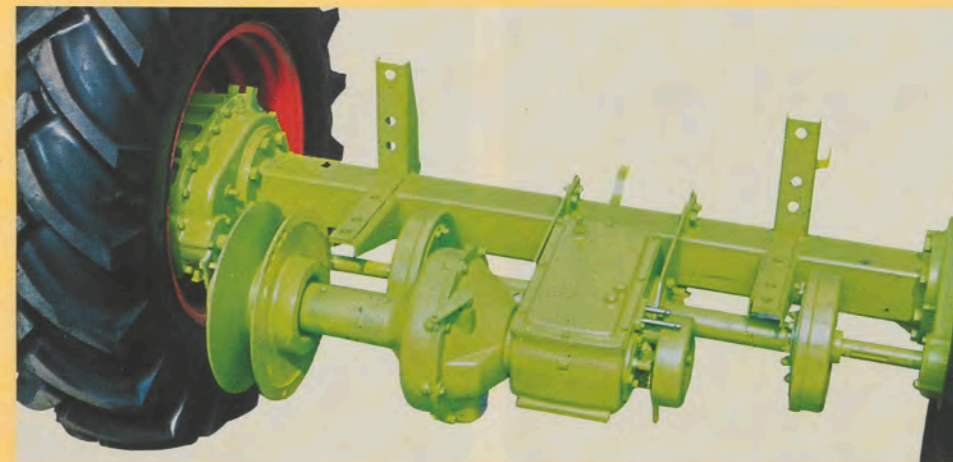
Robuste Antriebsachse
