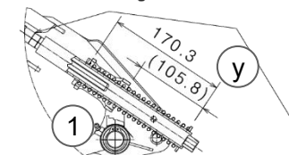
Einstellmaß fuer grossen Durchsatz
