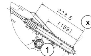
Einstellmaß fuer kleinen Durchsatz (Werkseinstellung)
