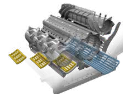
▲ Segmenty predného koša a segment hlavného koša môžu byť rýchlo vymenené.
