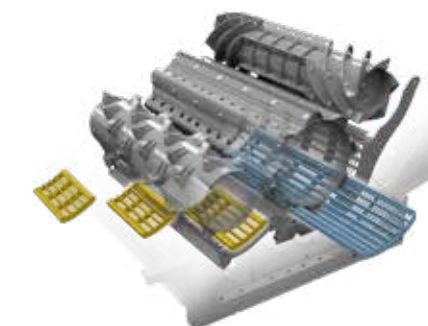
▲ Segmenty předního koše a segment hlavního koše mohou být rychle vyměněny.
