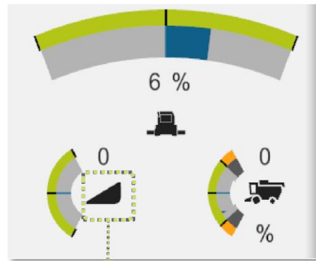
Feldfahrt mit leichter Querneigung und ohne Längsneigung
