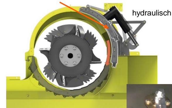
bewegliches Rotorleitblech
