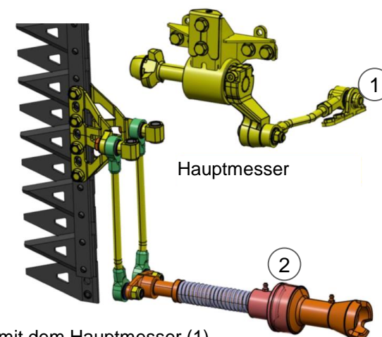
Mechanischer Antrieb der Seitenmesser über Koppelung mit dem Hauptmesser (1). Absicherung der Seitenmesser bei Überlast über den Kupplungsflansch und der Kupplungskugel (2).
