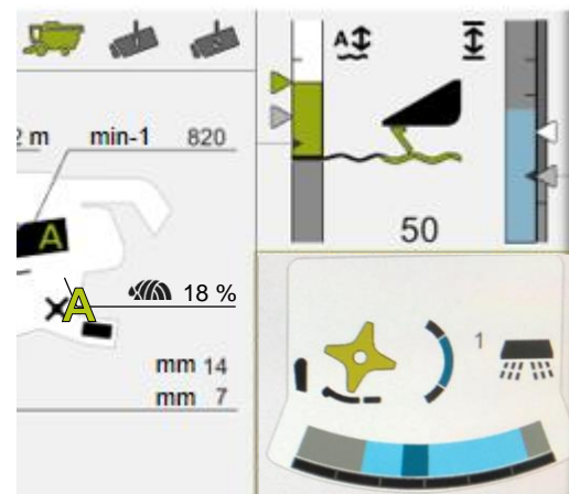
Anzeige der Häckslereinstellungen im CEBIS
