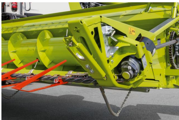
Halmteiler abnehmen und Einstellplatte über Camlock abnehmen.
