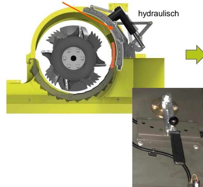
bewegliches Rotorleitblech
