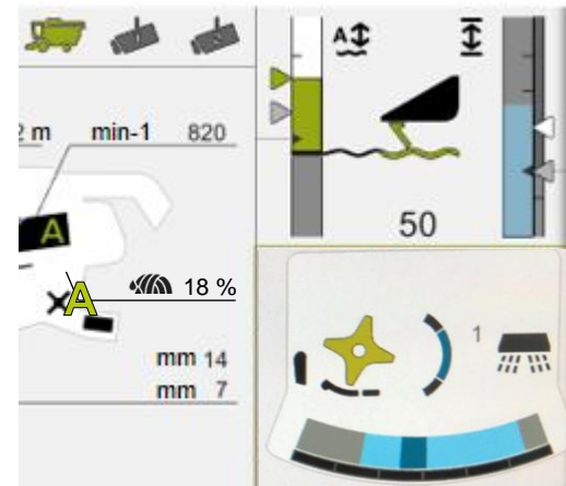
Anzeige der Häckselereinstellungen im CEBIS
