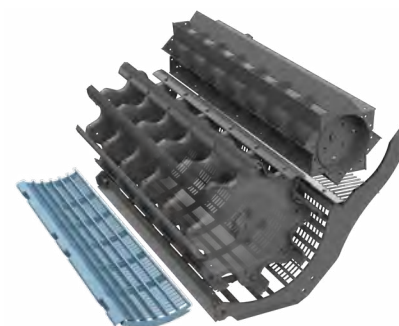
▲ Wymienny segment klepiska w modelu EVION 400.
