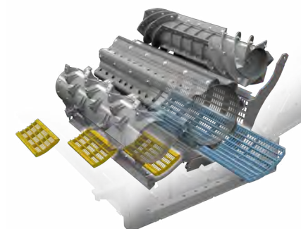
▲ Możliwa jest szybka wymiana segmentów klepiska wstępnego i segmentu klepiska głównego
