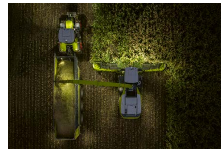
▲ Avec CLAAS connect, vous planifiez en amont les chantiers au bureau et vous les envoyez à la machine. Le conducteur n'a plus qu'à démarrer le chantier sur le CEMIS 1200. Page 48
