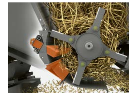
Gegenmesser und schwenkbares Bodenelement im SPECIAL CUT Häckslern
