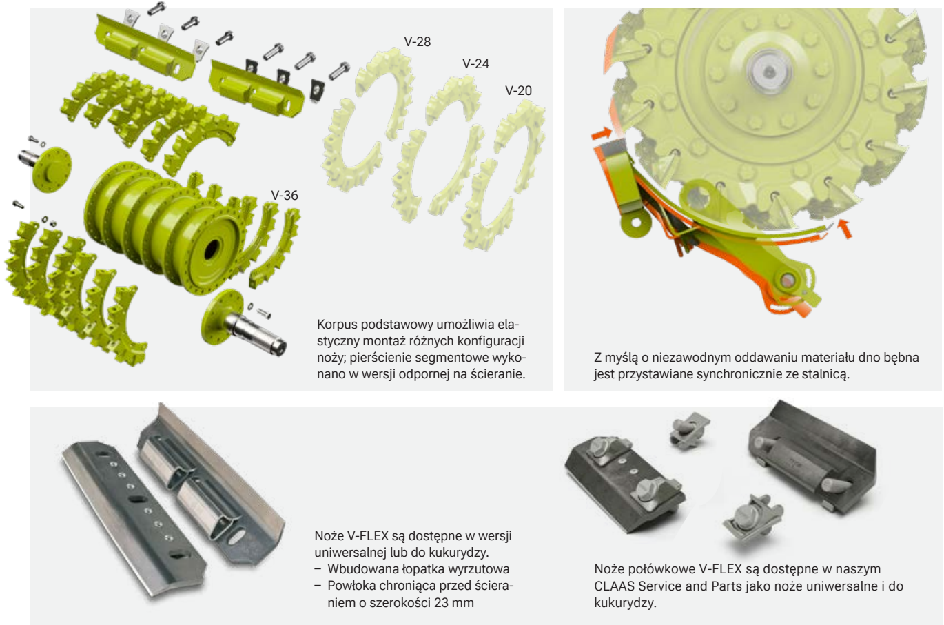
Długości cięcia bębnow nożowych.
