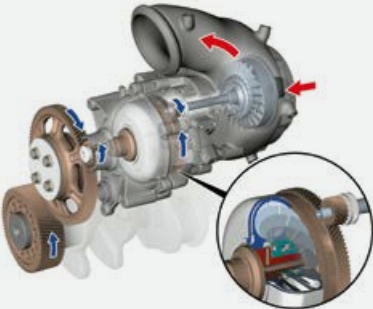
Turbo-Compound per OM 473 LA
