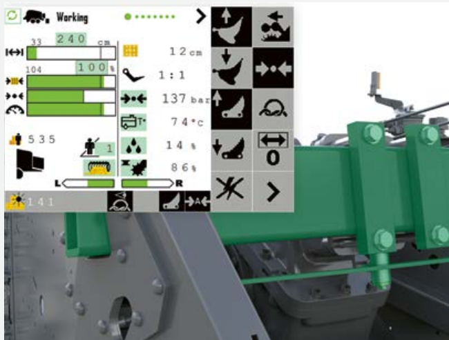
Die automatische Pressdruckregelung erfasst und visualisiert die Belastung der Pressenrahmen.
