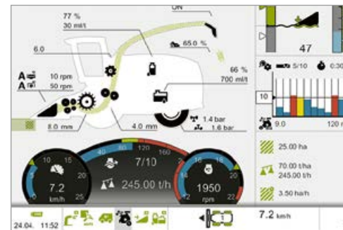
Распознавание состояния ножей с помощью индукции магнитного поля
