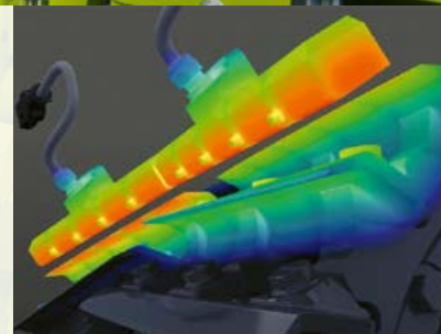
Распознавание состояния ножей с помощью индукции магнитного поля
