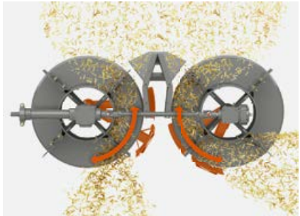
Esparcidor radial para un eficiente reparto de la paja con una mínima necesidad de fuerza
