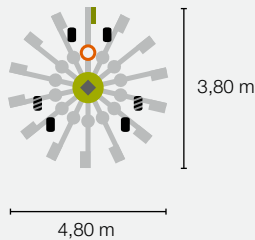
LINER 500 PROFIL
