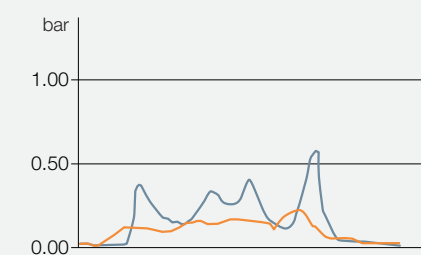
TERRA TRAC zonder kopakkerpositie
