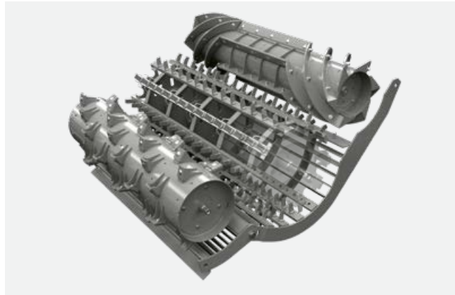
Das Reisdreschwerk oder der Umrüstsatz bestehen aus einer offenen Stiffentrommel und einem Stiffenkorb.
