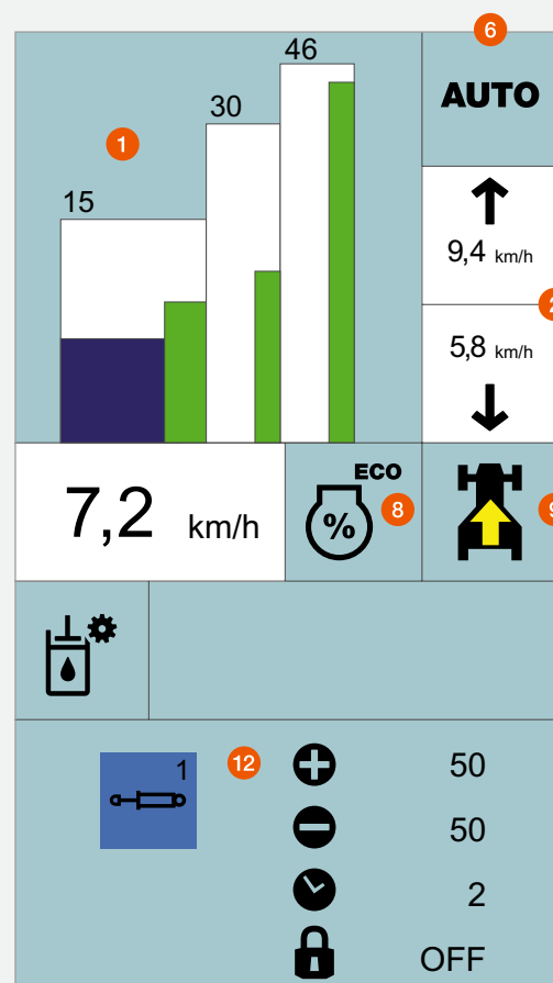
Écran couleur du CIS avec transmission CMATIC et menu de réglages sélectionné.
