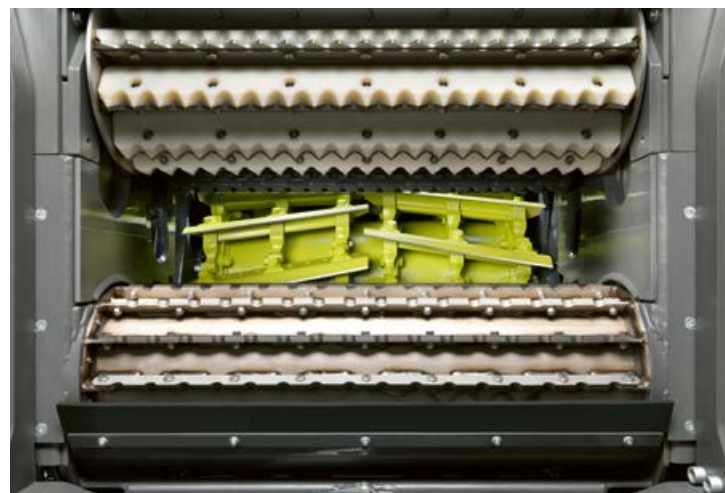
▲ El flujo de material adaptado al sistema – con hasta 910 mm, el más ancho del mercado – se encarga de un caudal un 20% mayor en todas las longitudes de picado. Página 22
