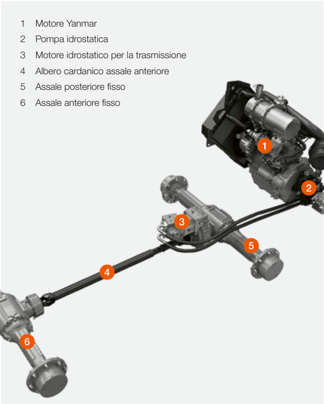
Trasmissione idrostatica con azione frenante autobloccante.
