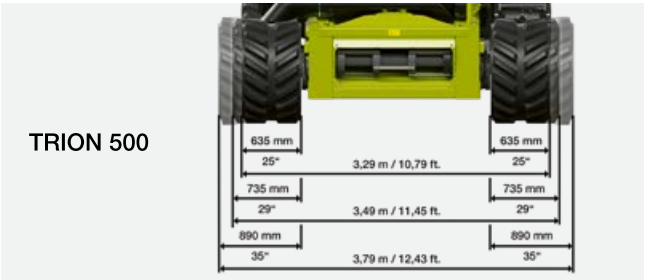
Cu șenilele de 635 mm, TRION devine mai îngust pe șosele, sporindu-vă mobilitatea.
