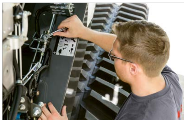
Treskeverkets turtallsområdene kan skiftes manuelt ved hjelp av en hydraulisk ventil.
