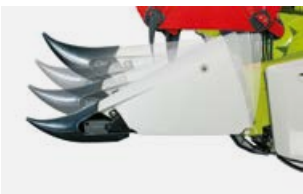
Diviseurs courts pour soja escamotables vers le haut
