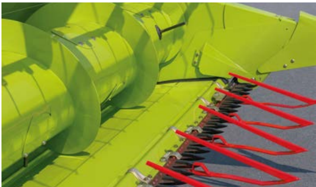
Tablier de coupe rentré – mode céréales ( -100 mm)
