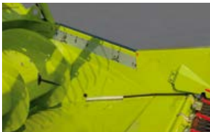
Marqueur de position du tablier de coupe parfaitement visible depuis la cabine
