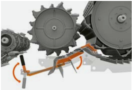
Klaffene i forbroen bidrar til å rense kornet.
