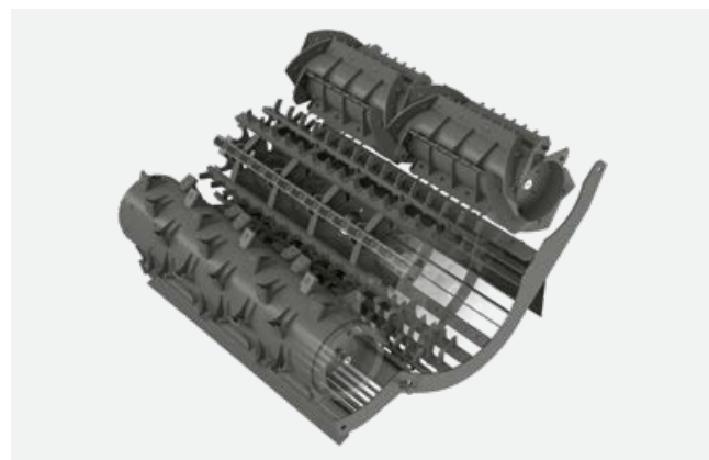
Ristærsekeværket eller ombygningssættet består af en åben pigcylinder og en pigbro.
