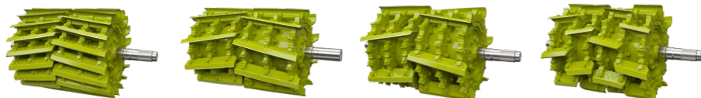
Полная установка ножей для короткой и средней длины резки.
