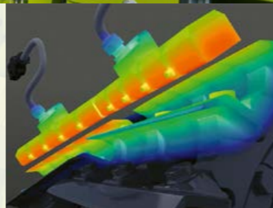
Reconocimiento del estado de cuchillas a través de la inducción del campo magnético
