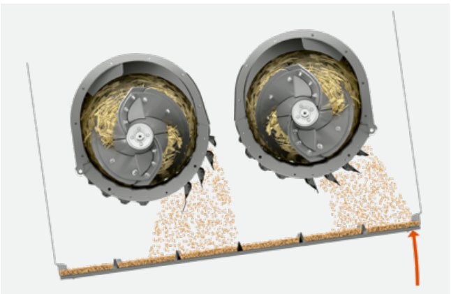
Potente limpieza 4D. El rendimiento de limpieza se mantiene constante también en terrenos desnivelados. 4D regula automáticamente la posición de las trampillas del rotor y apoya de forma activa al operario en un segundo plano.
