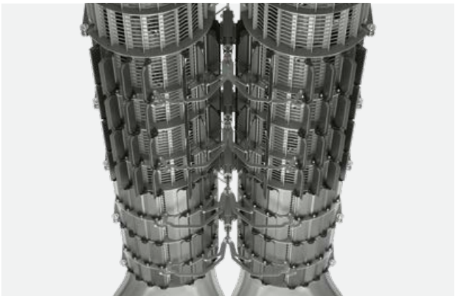
Reglaje hidráulico de las trampillas del rotor. Puede adaptar de forma variable la superficie de separación secundaria en CEBIS. Trampillas hidráulicas del rotor cierran hasta cuatro segmentos del rotor durante el avance.
