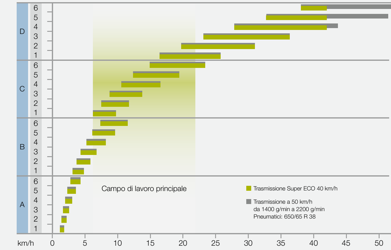
HEXASHIFT: 24 marce per scalare in modo ottimale
