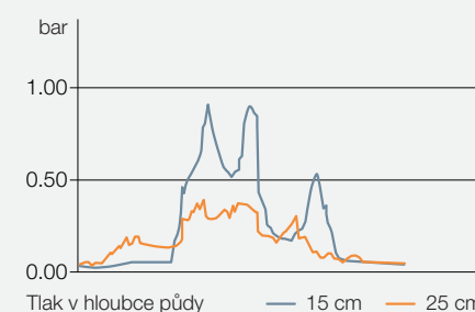
TERRA TRAC s ochranou souvrátí
