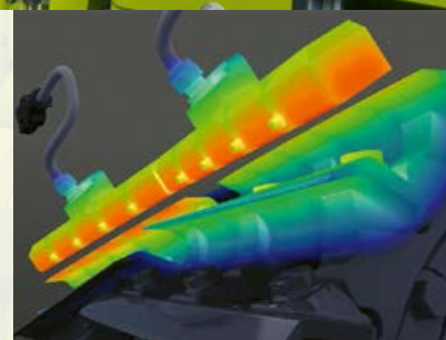
Detekce stavu nože pomocí indukce magnetického pole
