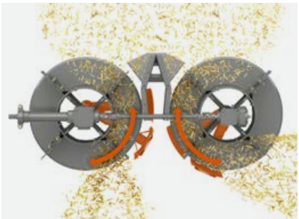
Împrăștiător radial pentru distribuția eficientă a paielor, folosind putere minimă
