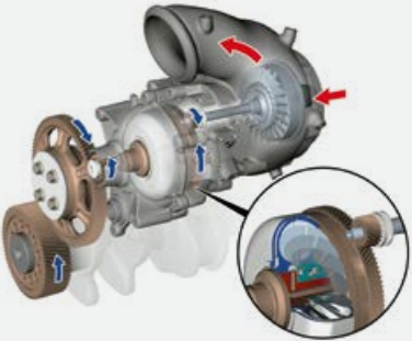
Turbo-Compound för OM 473 LA
