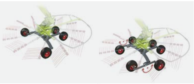
Guida ideale dei denti: grazie al carrello posizionato il più vicino possibile alla traiettoria dei denti.
