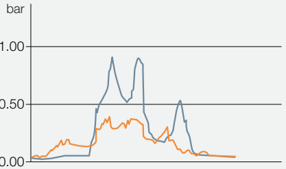
TERRA TRAC mit Vorgewendeschonung
