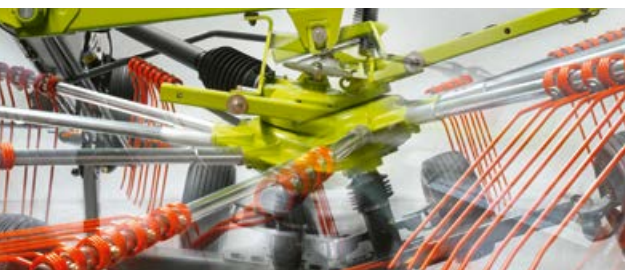
Enganche cardánico de los rotores: Los rotores se adaptan al suelo – independientemente del tractor.
