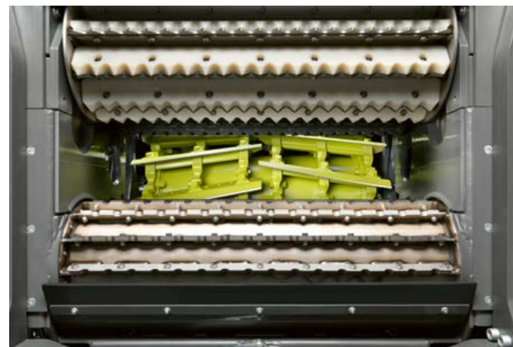
▲ Der systemabgestimmte Gutfluss – mit bis zu 910 mm der breiteste auf dem Markt – sorgt für 20% mehr Durchsatz in allen Häcksel-längen. Seite 22
