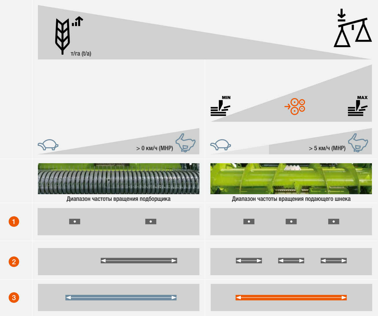
Частота вращения PICK UP. Варианты комплектации
