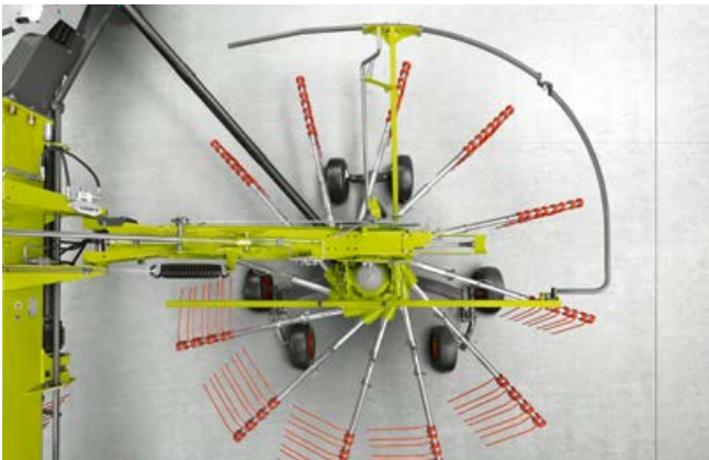
Гидравлические ограничители на разворотной полосе.
