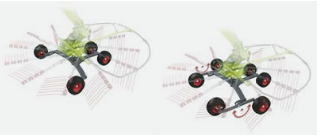
Идеальное направление пальцев: благодаря ходовой части ротора, которая расположена максимально близко к пальцам по периметру.
