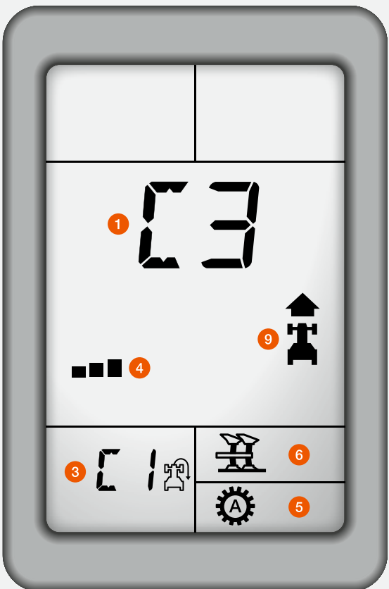
CIS display i instrumentpanelet og indikator for HEXASHIFT på A-stolpen.
