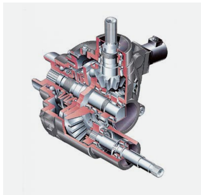
Vedligeholdelsesfri sikkerhed: Førsteklasses koblinger, der løber i oliebad, beskytter QUADRANT effektivt mod overbelastning.
