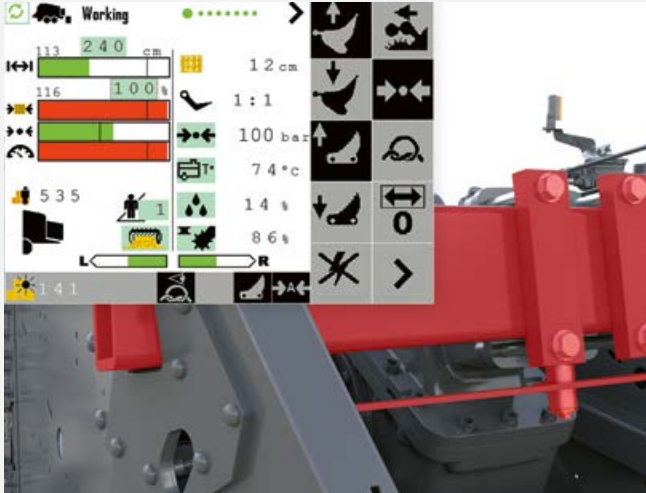
Sensoren på hovedrammen måler det udøvede pressetryk. Føreren får vist de målte værdier på CEMIS 700, og systemet regulerer belastningsgrænserne i overensstemmelse med disse værdier.
