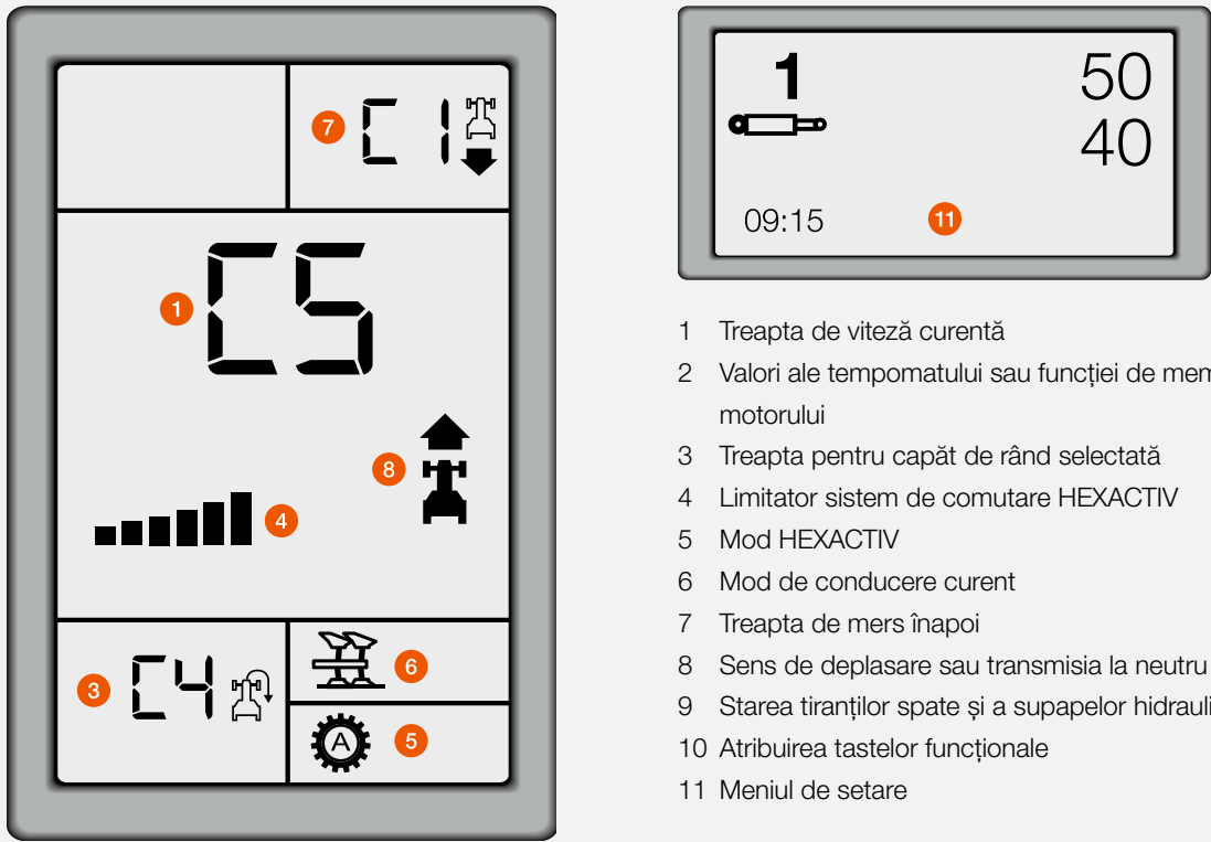
Afișaj CIS pe panoul de instrumente și afișaj pentru transmisie pe montantul A.
