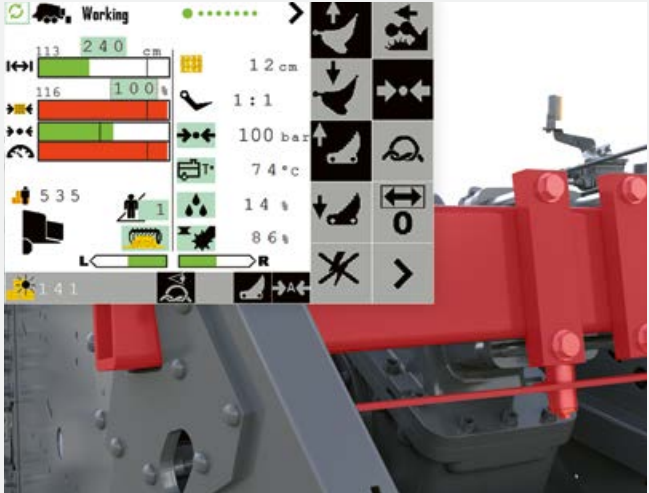
El sensor en el chasis principal mide la presión de empacado ejercida. Al operario le son mostrados los valores de medición en CEMIS 700. El sistema regula los límites de carga en base a estos valores.
