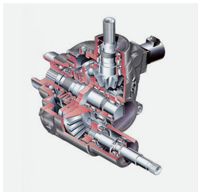
Bezobsługowe bezpieczeństwo: mocne, pracujące w kąpiel olejowej sprzęgło doskonale chronią QUADRANT przed przeciążeniami.
