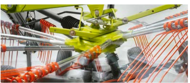
A kardáncukkos rotorfelfüggesztés biztosítja a rotorok traktortól független talajkövetését.
