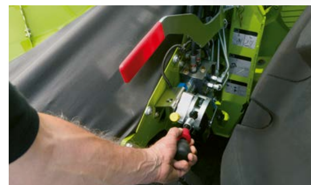
Padeves trumuļu ātruma regulēšana trīs pakāpēs – optimālai augu masas plūsmi.
