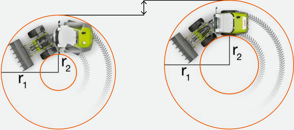
TORION SINUS su vairuojamu galiniu tiltu
