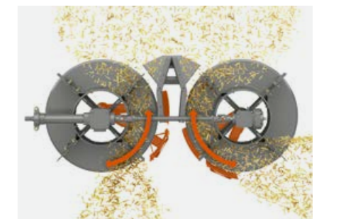
POWER SPREADER ger effektiv fördelning av hackad halm med minimalt effektbehov.
